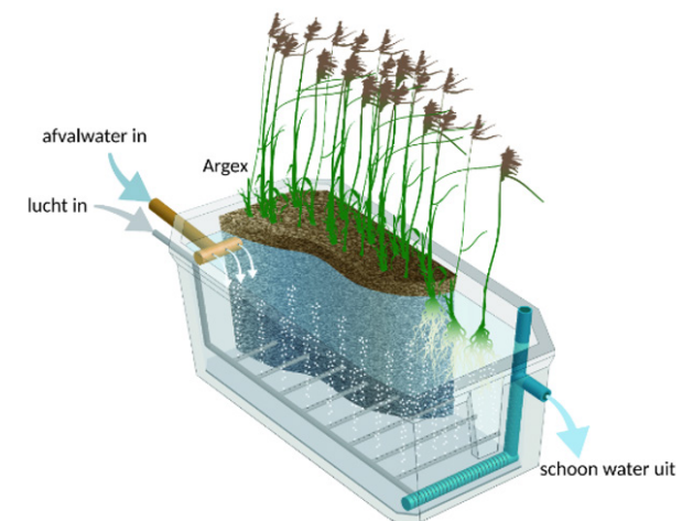
Figuur 28 Phytocube, de compacte oplossing. Bron: Rietland
