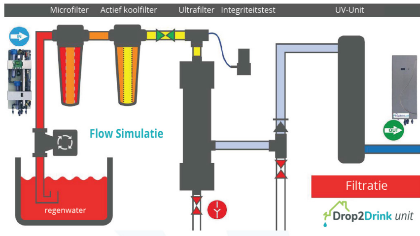
Figuur 16 Drop2Drink Unit die hemelwater zuivert tot drinkwaterkwaliteit. Bron: D2D Water Solutions
